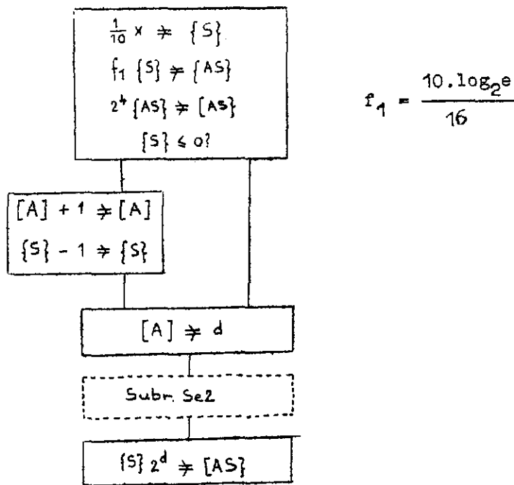
Blokschema e^x = [AS] als |x| < 10 .
